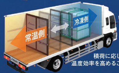
庫内を前後に分け 温度帯別の商品管理が可能
