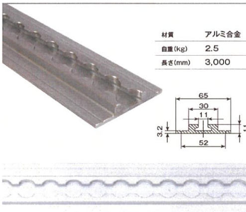
品番：JM-AR-M-F エアラインレール®中量用(フランジ付き)
