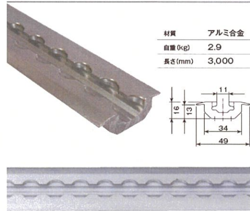
品番：JM-AR-S エアラインレール®重量用(埋め込みタイプ)
