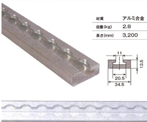
品番：JM-AR-HA エアラインレール®重量用
